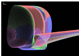
Расчетная сетка на поверхности модели
