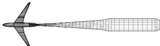
Расчетная сетка для комбинации модели и килевой державки
